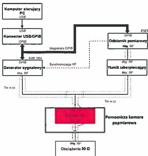
Rys. 1. Schemat blokowy układu pomiarowego do pomiaru tłumienności filtrów (pomiar odniesienia)
