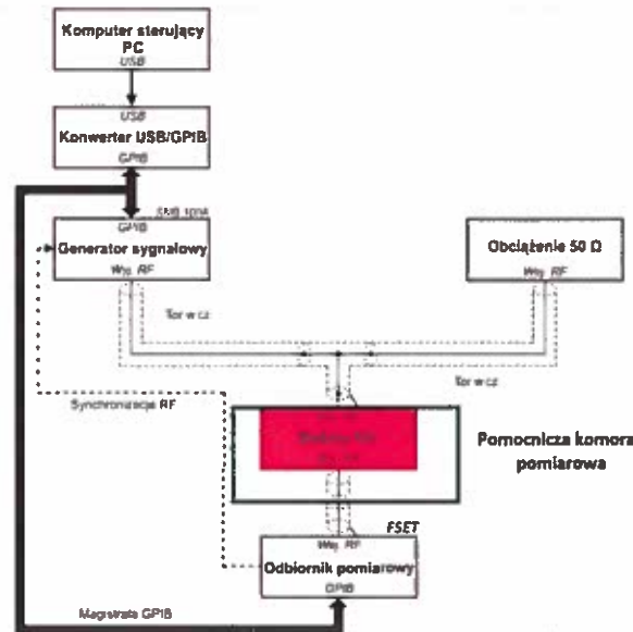
Rys. 2. Schemat blokowy układu pomiarowego do pomiaru tłumienności filtrów (pomiar zasadniczy)
